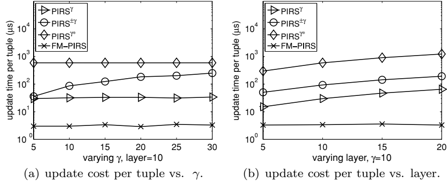
Fig. 4. \text{PIRS}^\gamma , \text{PIRS}^{\pm\gamma} , \text{PIRS}^{\gamma*} , FM-PIRS: update cost.
